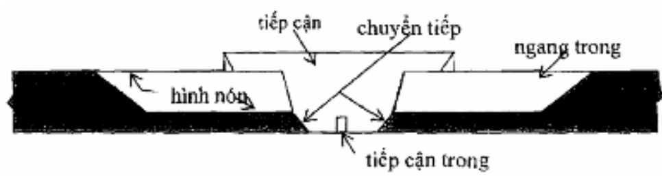
Mặt cắt B - B
