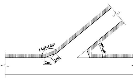
Kích thước vật góc tại góc cắt giao nhau với lộ giới từ 140^\circ đến dưới 160^\circ
