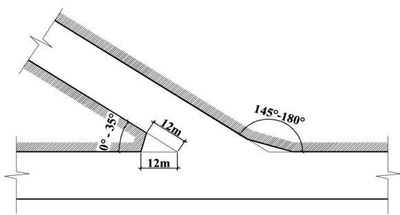
Kích thước vật góc tại góc cắt giao nhau với lộ giới nhỏ hơn 35^\circ
