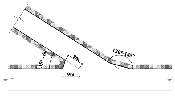
Kích thước vật góc tại góc cắt giao nhau với lộ giới từ 35^\circ đến dưới 60^\circ
